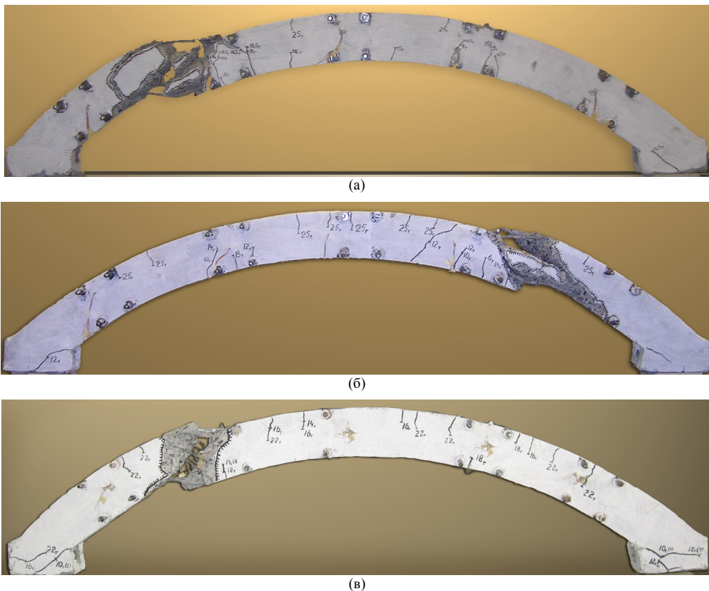
Рис. 7. Характер руйнування арок: (а) – 1А-1, (б) – 1А-3, (в) – 2А-4
