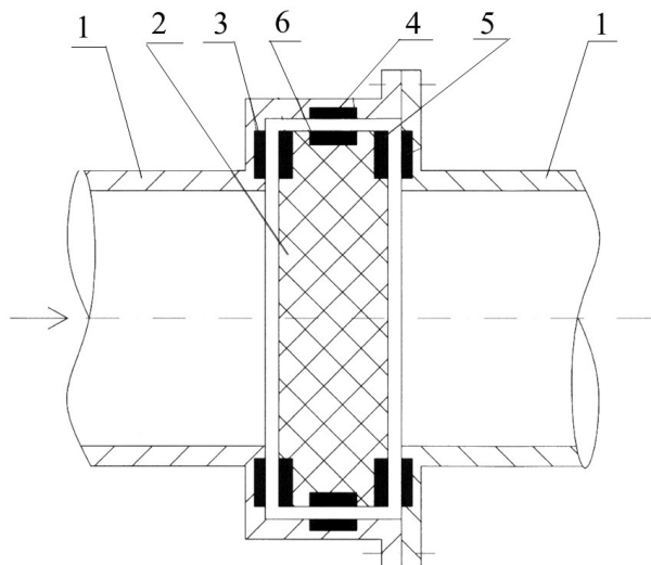
Рис.1. Схема лічильника безопорного
