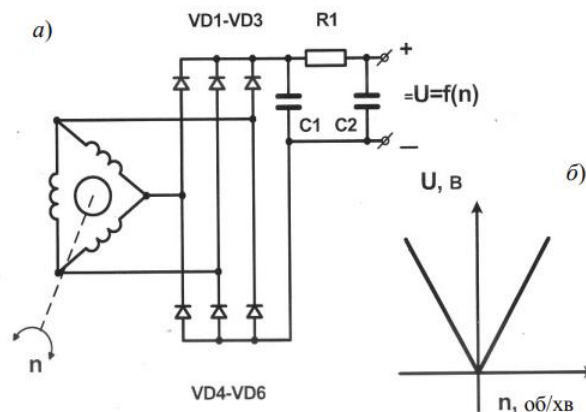
Рисунок 5.7 – Синхронний тахогенератор змінного струму
