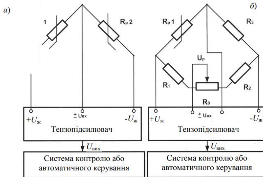
Рисунок 3.6 – Схеми відімкнення тензометричних датчиків
