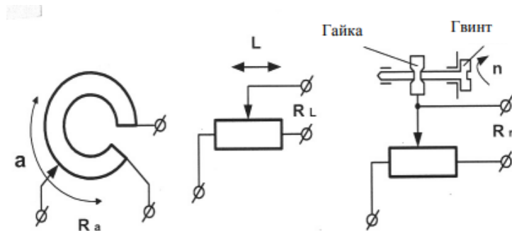
Рисунок 3.1 – Основні конструкції потенціометричних перетворювачів
