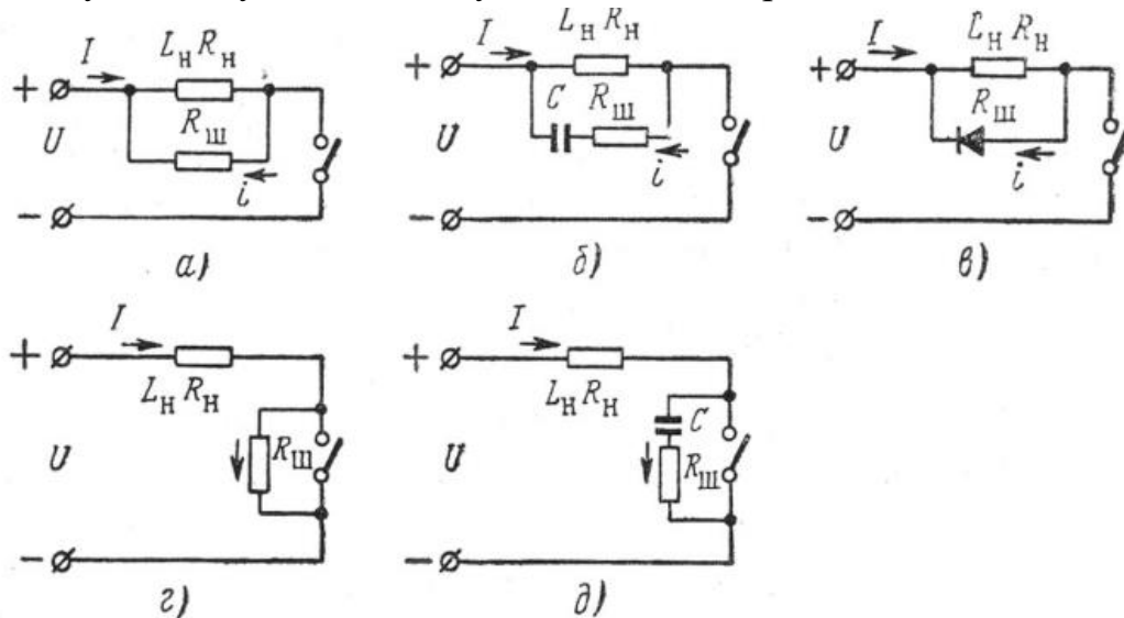
Рисунок 6.4 – Схеми іскрогасіння
