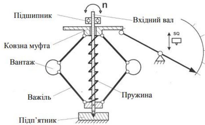
Рисунок 5.2 – Відцентровий тахометр
