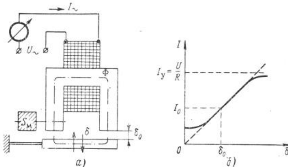
Рисунок 3.11 – Індуктивний давач
