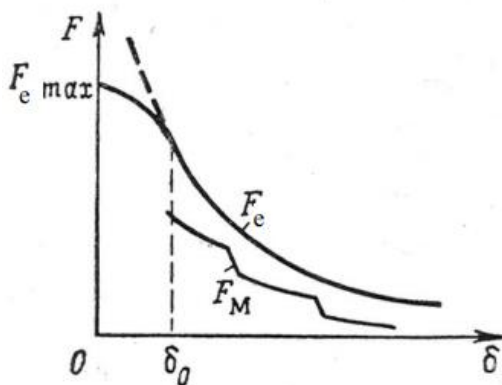
Рисунок 6.3 – Електромеханічна та механічна характеристики реле
