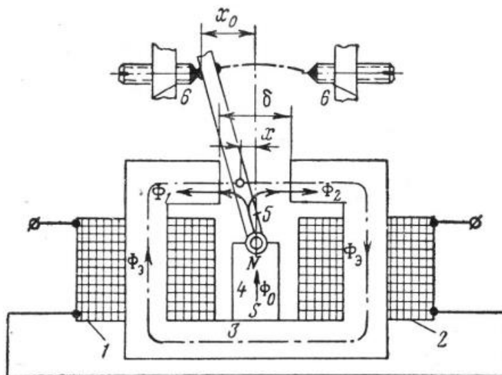
Рисунок 6.5 – Поляризоване реле:
