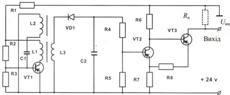
Рисунок 3.16 – Принципова електрична схема безконтактних кінцевих вимикачів БК-А, ВКБ, КВД
