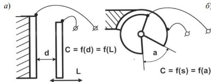
Рисунок 3.20 – Ємнісні перетворювачі для вимірювання лінійних та кутових переміщень
