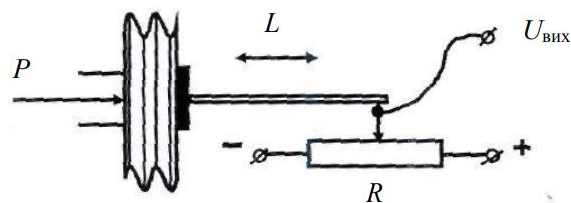
Рисунок 1.3 – Схема давача тиску
