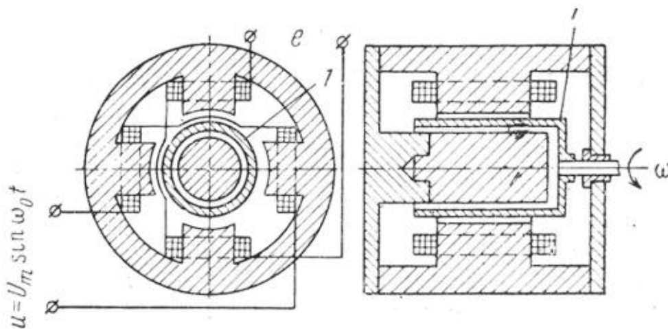
Рисунок 5.6 – Конструкція двофазного асинхронного тахогенератора
