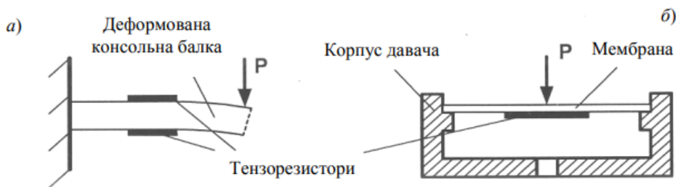
Рисунок 3.5 – Встановлення тензорезисторів
