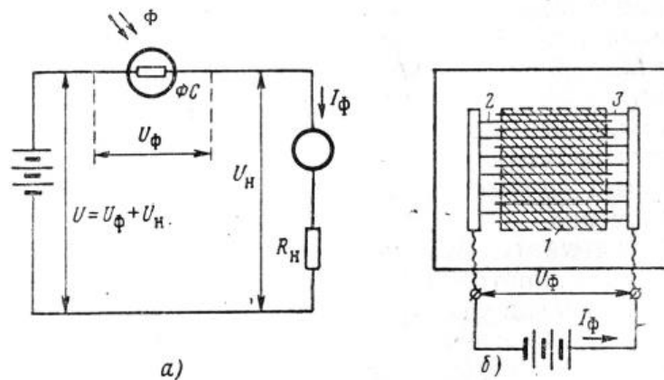
Рисунок 3.10 – Схема увімкнення (а) і конструкція (б) фоторезистора
