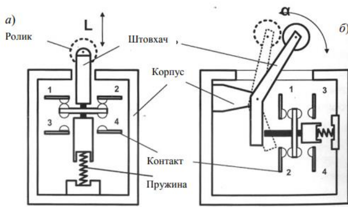
Рисунок 4.1 – Конструкції кінцевих вимикачів нажимної та повертальної дії
