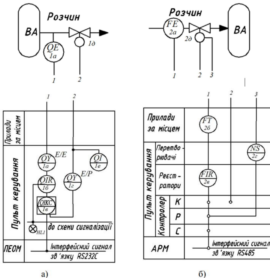
Рисунок 7.2 – Функціональні схеми САУ, реалізованих з використанням мікропроцесорних регуляторів (а) та контролера (б): ВА – випарний апарат; К,Р,С – функціональні можливості контролера, відповідно контролю, регулювання, сигналізації; АРМ – автоматизоване робоче місце оператора.
