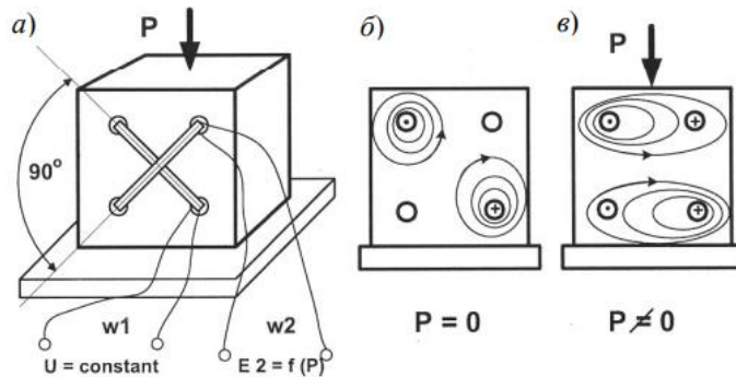
Рисунок 3.14 – Магнітоанізотропний перетворювач
