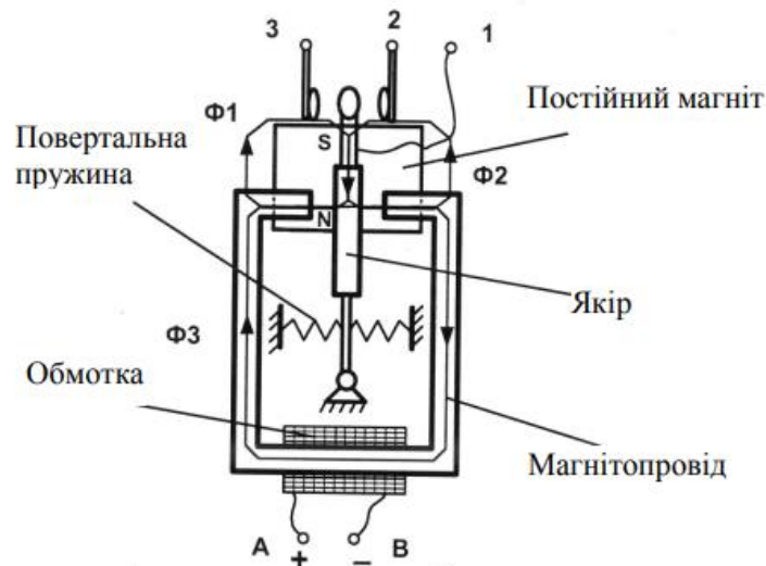
Рисунок 6.6 – Конструкція полярного реле
