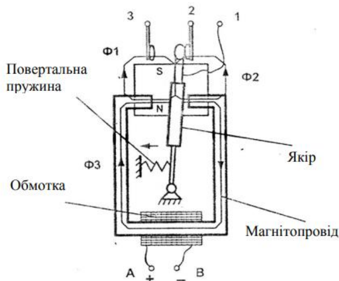
Рисунок 6.7 – Двопозиційне полярне реле
