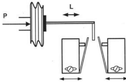
Рисунок 4.5 – Мікроперемикачі у складі давача тиску
