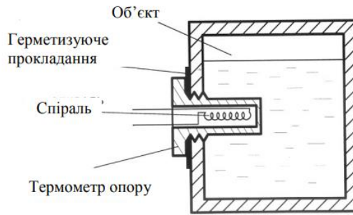
Рисунок 3.7 – Термометр опору
