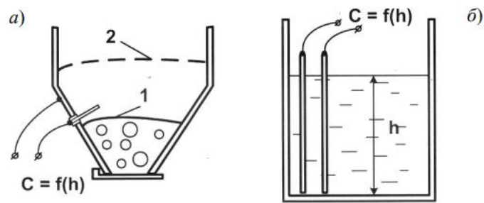
Рисунок 3.19 – Ємнісні давачі рівня
