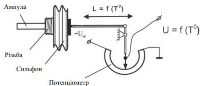
Рисунок 3.2 – Електричний термометр
