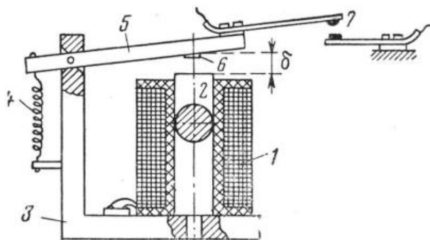
Рисунок 6.2 – Електромагнітне реле з поворотальним якорем
