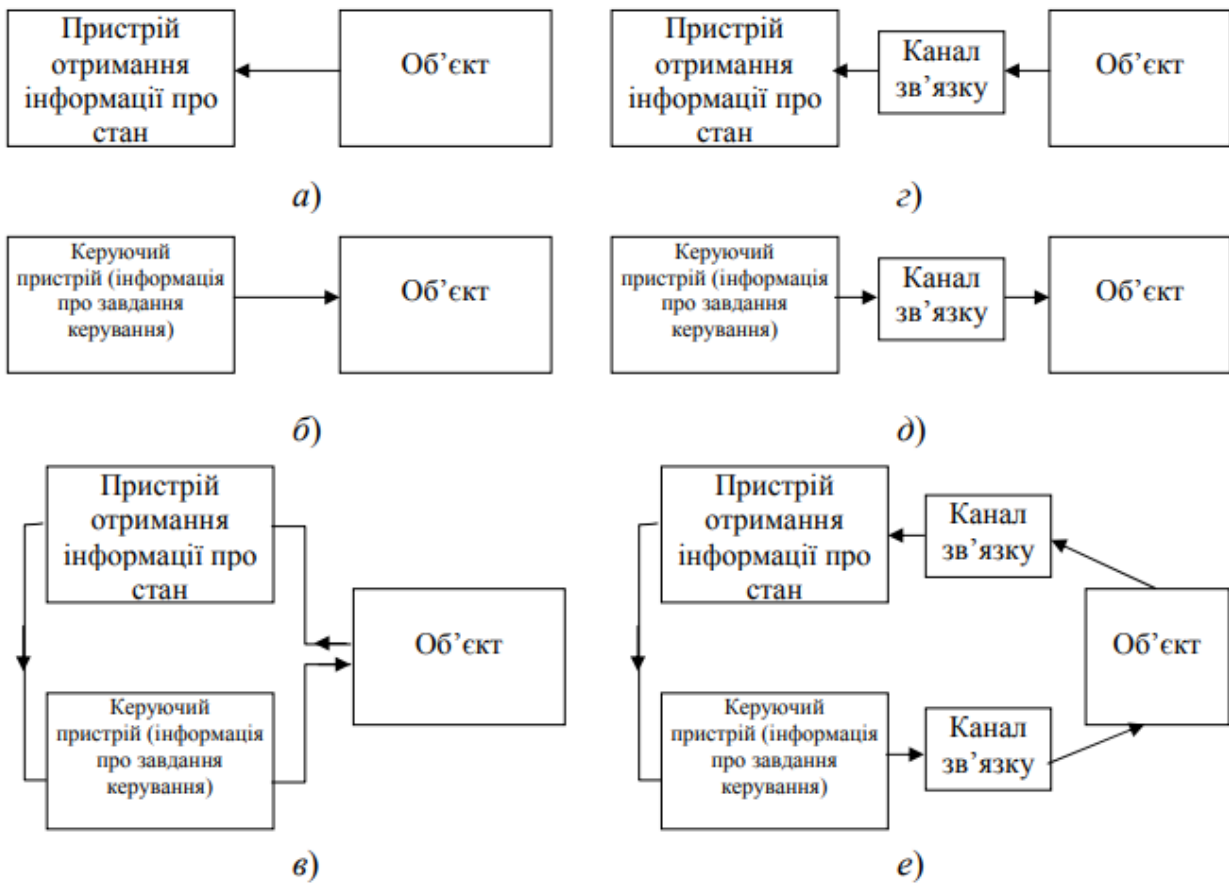
Рисунок 1.1 – Загальні схеми типових форм автоматизації
