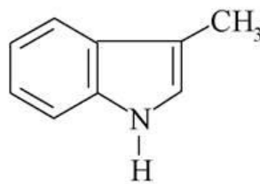
скатол
