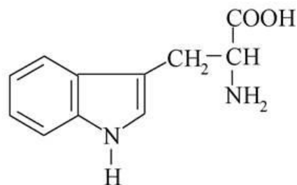
триптофан
