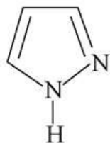
піразол
