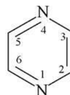
піразин
