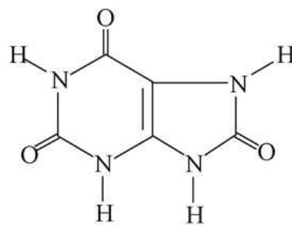
сечова кислота
