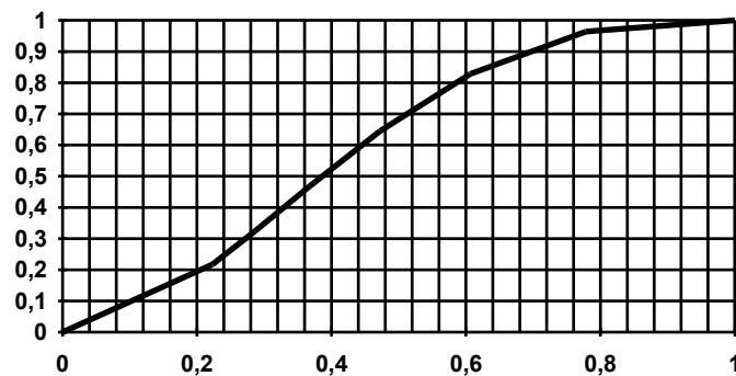
Рисунок 6 – Залежність ймовірності безвідмовної роботи системи «2 з 4» від ймовірності безвідмовної роботи її елементів.
