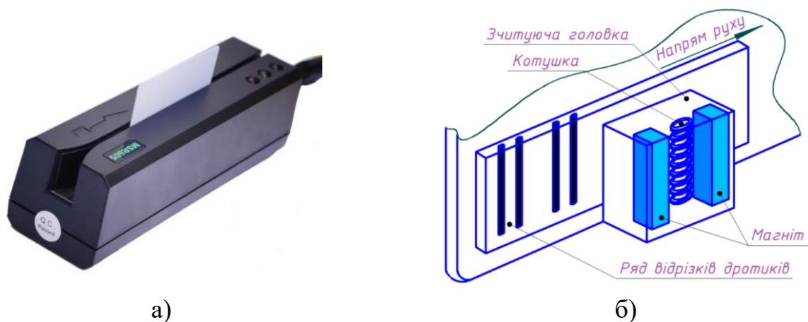
Рисунок 3.2 – Кардрідер [110]
