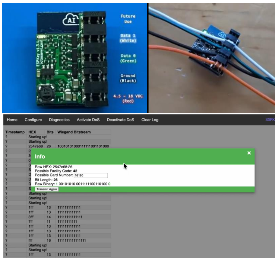
Рисунок 5.1 – Модуль BLEKey та вікно зчитування даних карти
