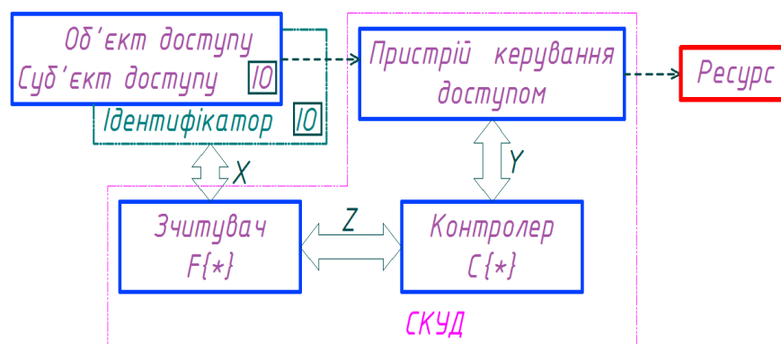
Рисунок 2.1 – Узагальнена структурна схема СКУД [110]
