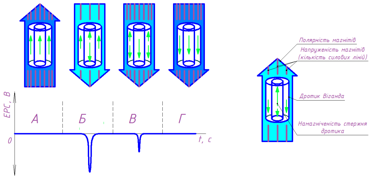
Рисунок 3.3 – Процес формування сигналів [110]
