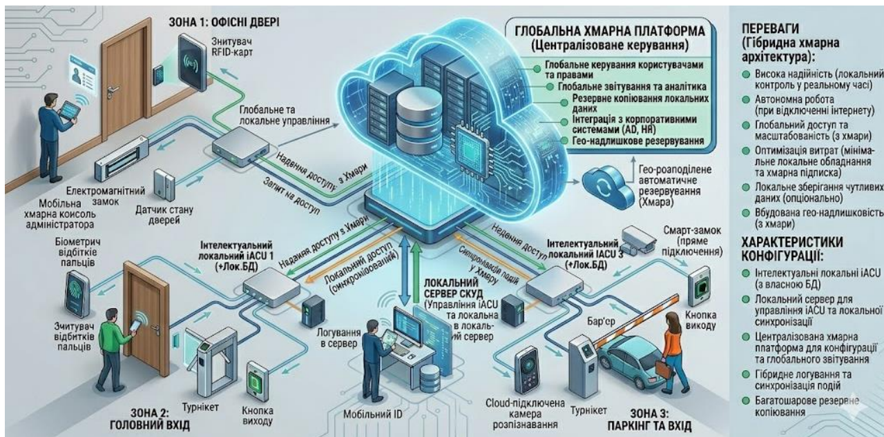
Рисунок 7.4 – Топологія гібридної хмарної архітектури
