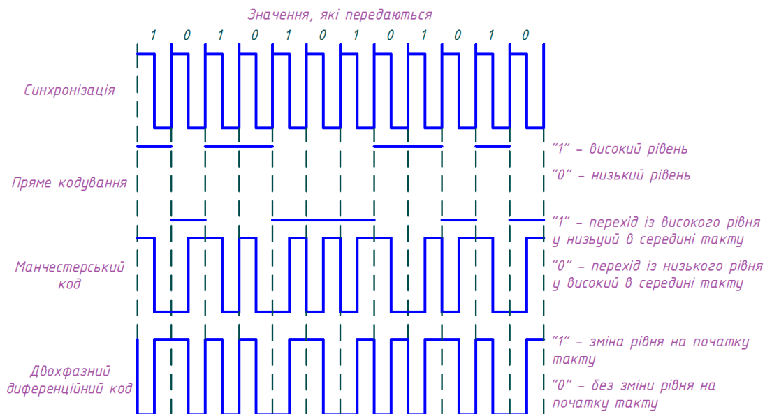
Рисунок 3.12 – Способи кодування даних [110]
