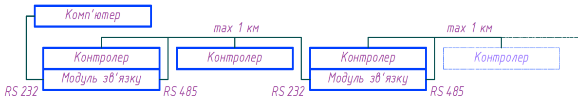
Рисунок 9.8 – Збільшення довжини гілки шляхом використання двох модулів зв'язку
