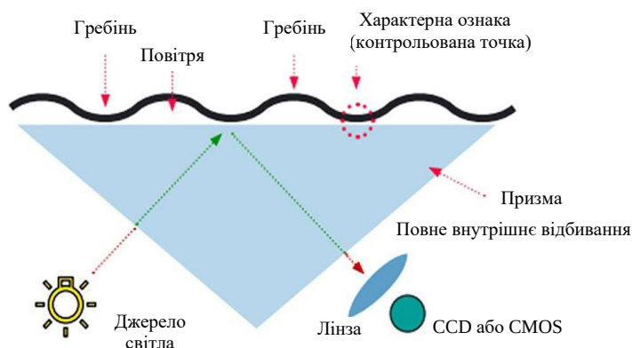
Рисунок 4.3 – Функціональна схема оптичного зчитувача відбитка пальця [110]
