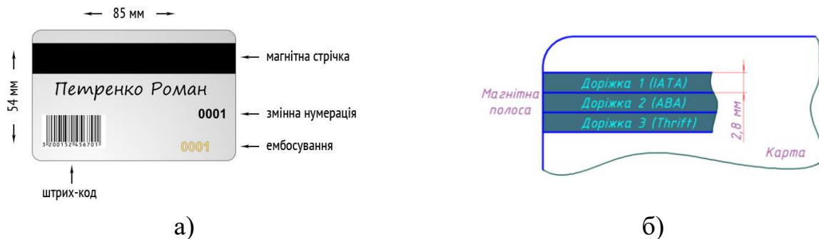
Рисунок 3.6 – Пластикова карта з магнітною стрічкою [110]
