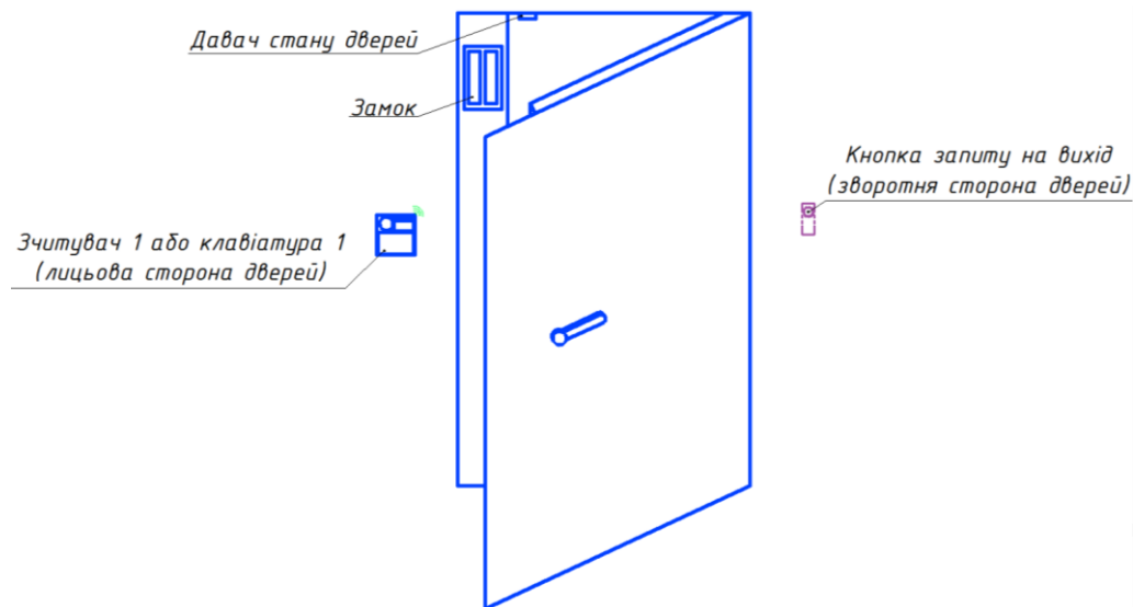
Рисунок 2.11 – Технічні засоби точки доступу з одностороннім контролем
