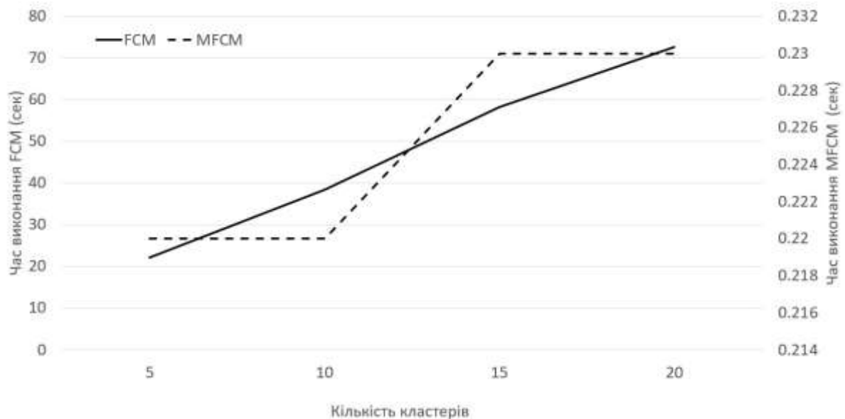
Рисунок 2 – Залежність часу виконання 100 ітерацій для програмної реалізації FCM та MFCM при зміні кластерів від 5 до 20 з кроком 5
