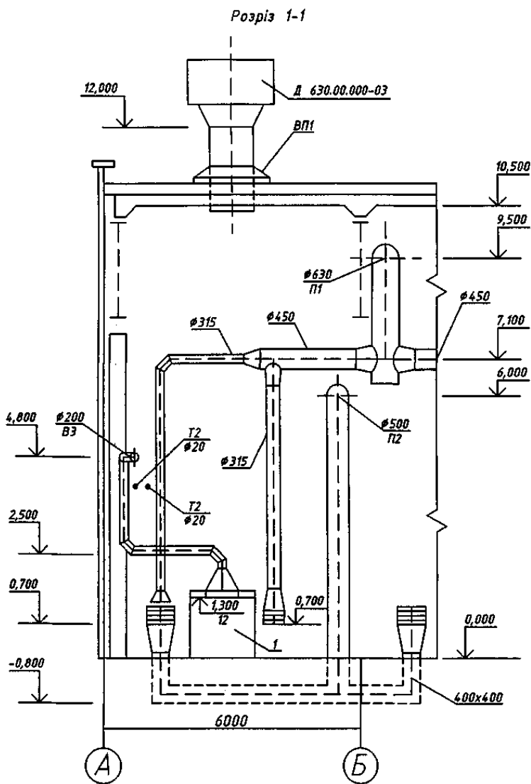
Рис. В.5. Приклад оформлення Розрізу 1-1 системи вентиляції будівлі
