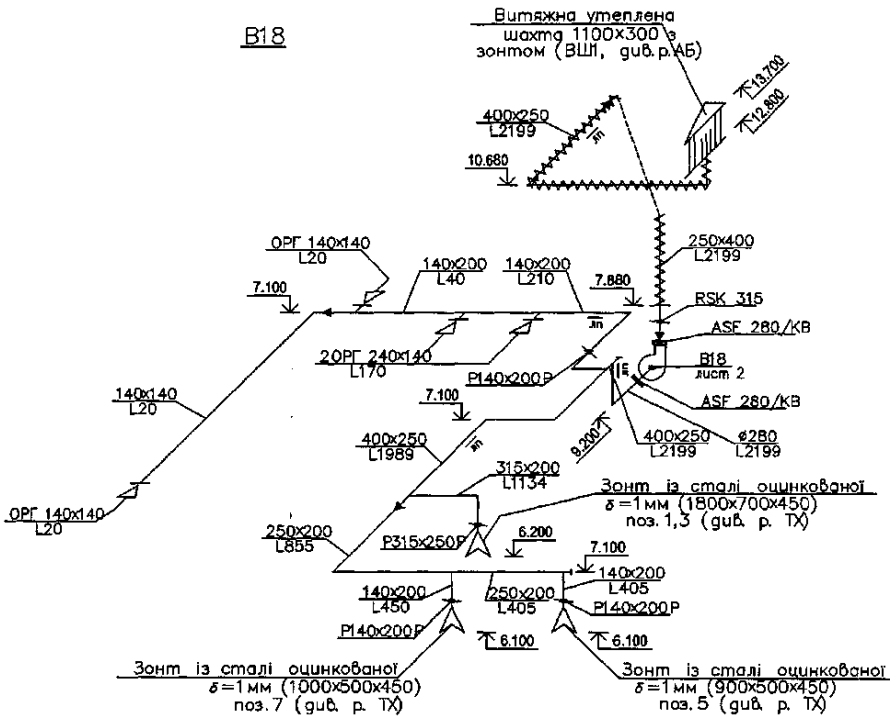
Рис. Г.8. Приклад оформлення аксонометричної схеми системи витяжної механічної вентиляції B18 будівлі
