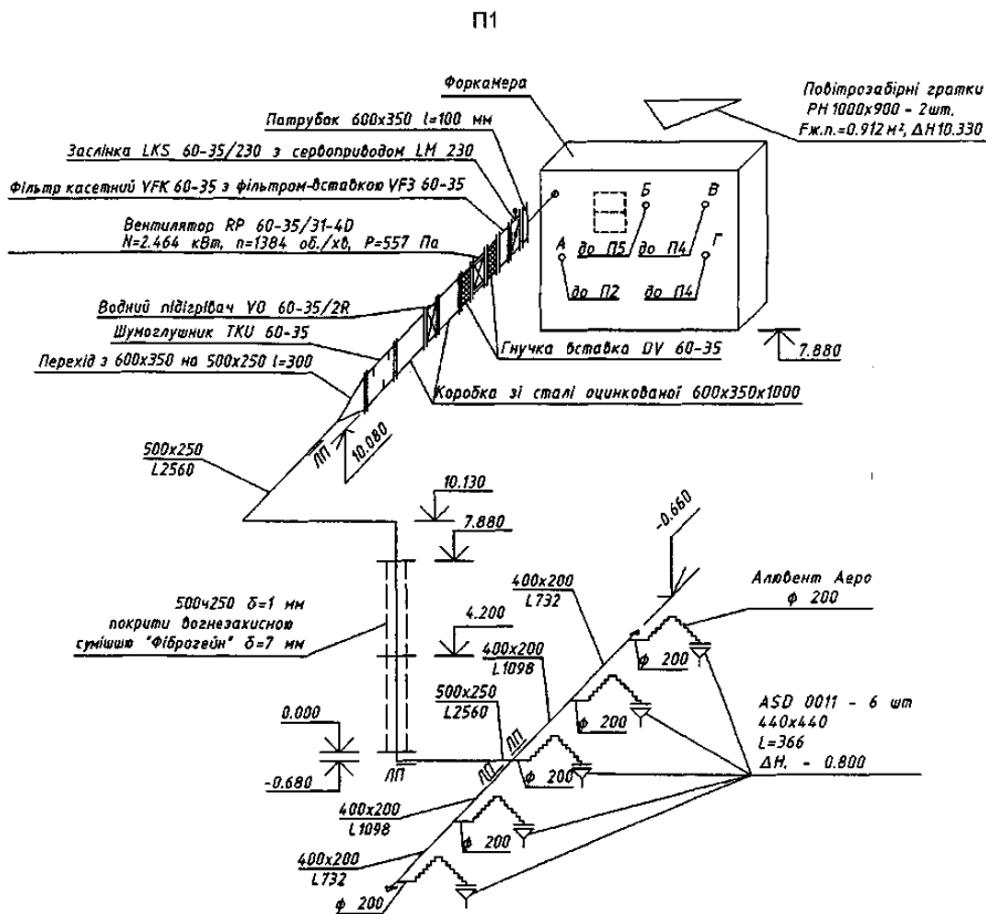
Рис. Г.7. Приклад оформлення аксонометричної схеми системи припливної механічної вентиляції П1 будівлі
