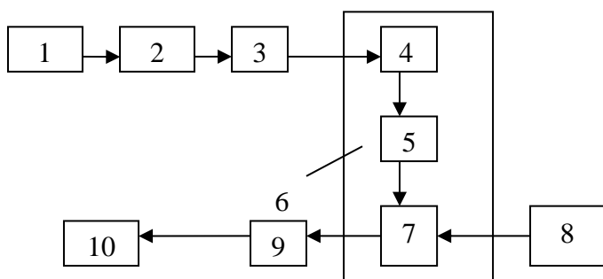
Блок-схема газорідинного хроматографа
