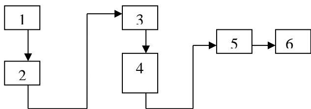
Принципова схема рідинного хроматографа 1-ємність для елюанта; 2-насос; 3-дозатор; 4-колонка; 5-детектор; 6-реєстратор.
