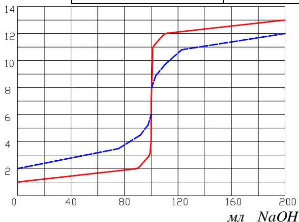
Рисунок 1. Криві титрування сильною кислотою сильною основою.
