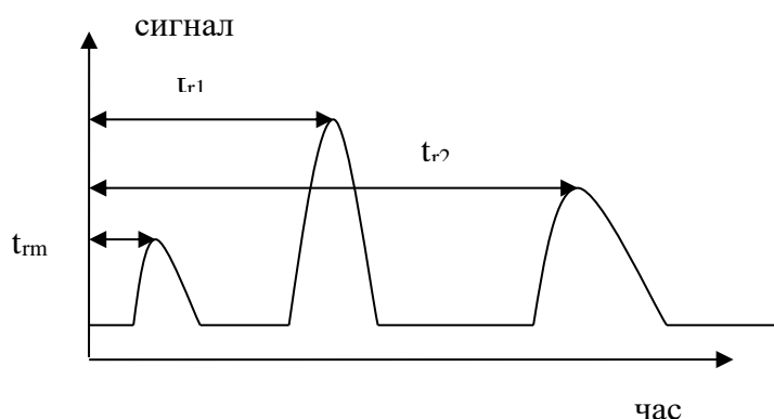
Хроматограма суміші двох речовин t_{rm} – час перебування речовин у рухомій фазі
