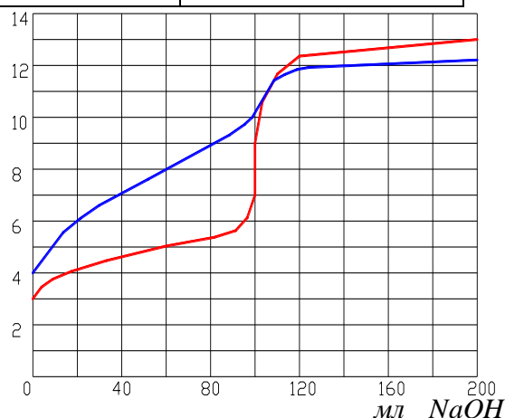
Рисунок 2. Криві титрування слабких кислот ( \text{CH}_3\text{COOH} і \text{H}_3\text{BO}_3 ) сильною основою (NaOH)
