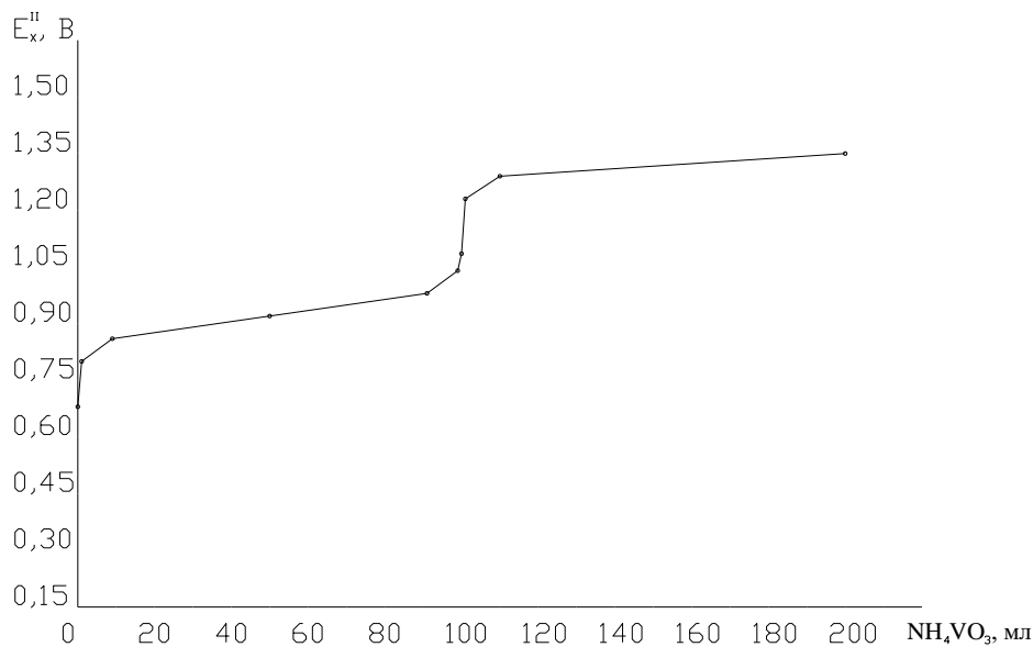
Крива титрування \text{FeSO}_4 в 10\text{N H}_2\text{SO}_4 розчином \text{NH}_4\text{VO}_3 .
