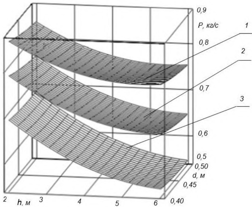
Рисунок 4.2 – Залежність продуктивності комбінованого забірною пристрою P від діаметру транспортуючого трубопроводу d та глибини розробки h , за швидкості занурення m : 1 – 0,3 м/с; 2 – 0,25 м/с; 3 – W=0,2 м/с
