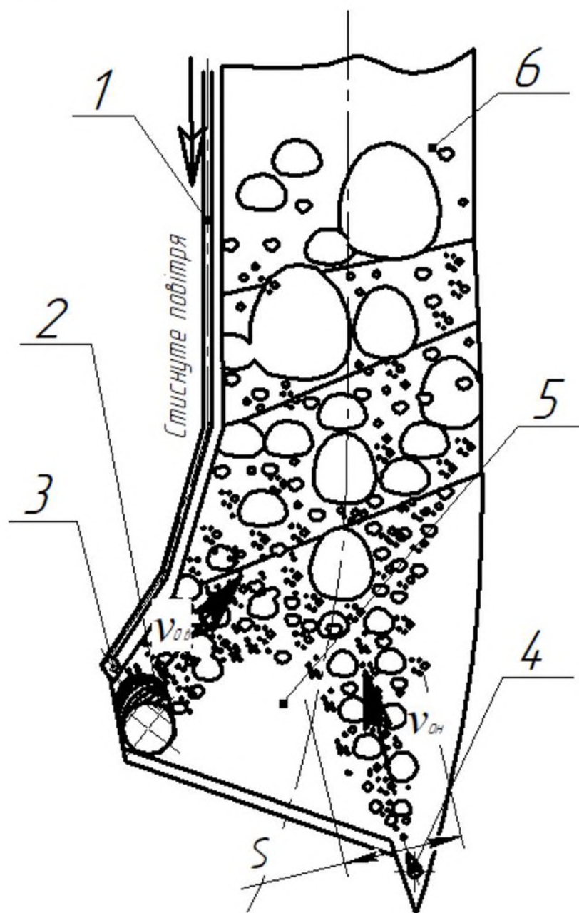
Рисунок 2.2 – Розрахункова схема дії потоку повітря на сапропель: 1 – повітрепровід, 2 – напірний верхній розпушувач, 3 – турбіна, 4 – нижній розпушувач з форсунками, 5 – корпус
