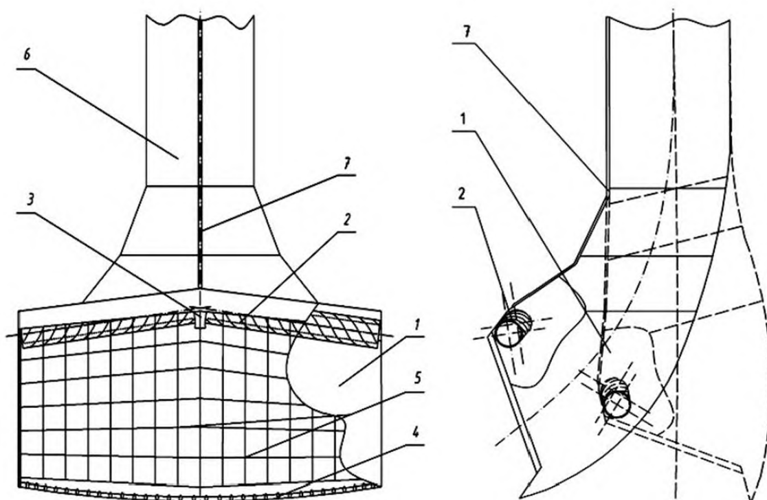
Рисунок 2.1 – Схема забірного пристрою: 1 – змішувач; 2 – напірний верхній розрихлювач; 3 – турбіна; 4 – нижній розрихлювач; 5 – захисна решітка; 6 – підйомний трубопровід; 7 – магістраль подачі повітря.
