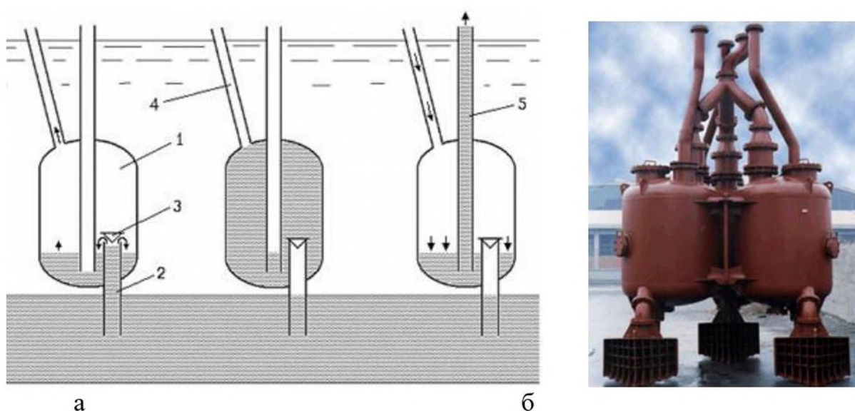
Рисунок 1.6 – Схема роботи (а) та фото пневматичного камерних насоса із всмоктуючим забірним пристроєм у формі ковша (б): 1 – робоча камера, 2 – всмоктуючий патрубок, 3 – вхідний клапан; 4 – труба подачі і скидання повітря, 5 – трубопровід подачі пульпи.
