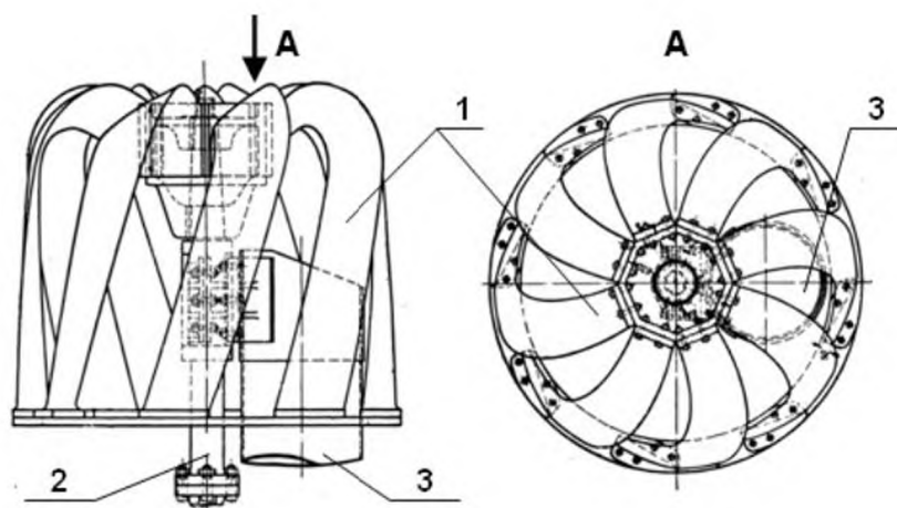
Рисунок 1.5 – Фрезерний забірний пристрій для добування зарослих донних покладів: 1 – торцева фреза; 2 – вал приводу; 3 – всмоктувальний трубопровід.
