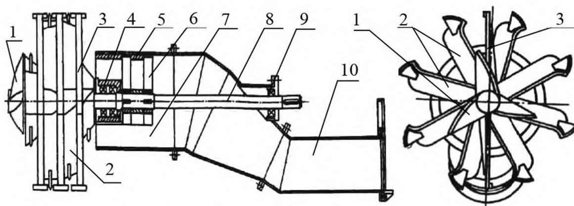
Рисунок 1.4 – Забірний пристрій з роторним розрихлювачем: 1 – фреза; 2 – ріжучий ніж; 3 – протиріжучий ніж; 4, 9 – опори; 5 – ніж статор подрібнювач; 6 – ніж ротор подрібнювач; 7 – всмоктувальний ркуав; 8 – вал; 10 – вивідний трубопровід.
