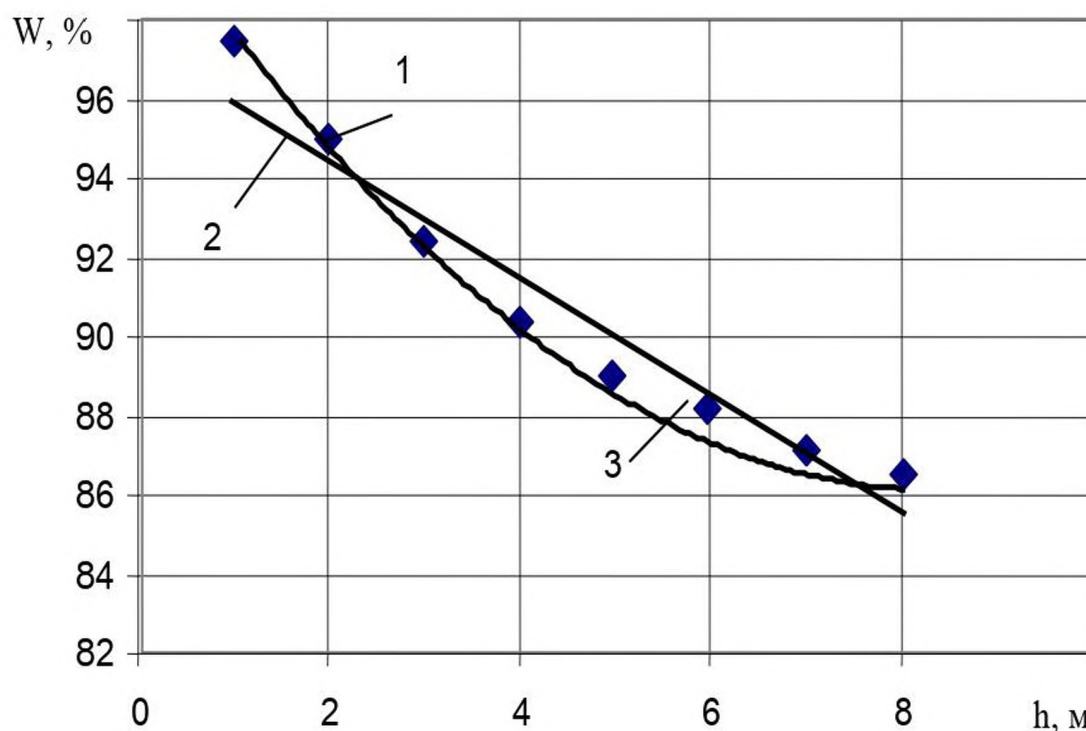
Рисунок 3.5 Залежність природної вологості органічного сапропелю W від глибини розміщення h : 1 – експериментальні точки; 2 – лінійна апроксимація; 3 – апроксимація поліномом другого порядку.
